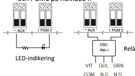
Exempel på inkoppling till PGM-utgång
