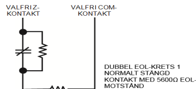
Dubbelbalanserade sektioner
