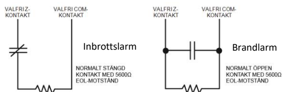
Enkelbalanserade sektioner
