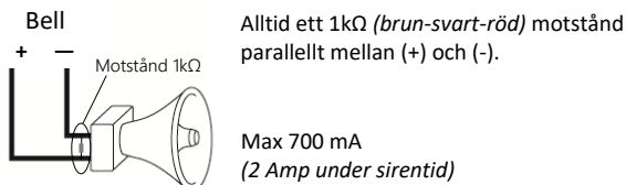
Inkoppling sirenutgång
